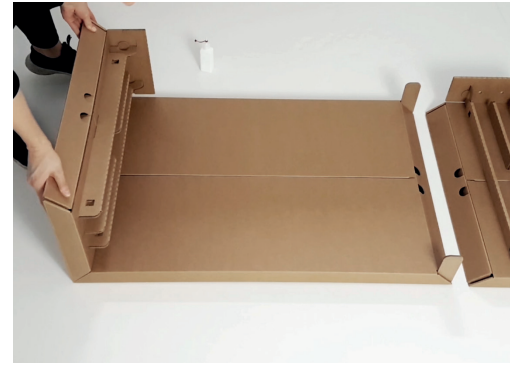
Seitenteil auf die Winkel schieben, bis die schrägen Flächen fest aufeinander sitzen
