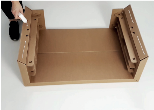
Auf die oberen schrägen Flächen auch etwas Leim auftragen
